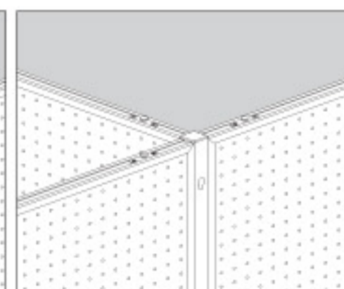
三方向連結(T字)
