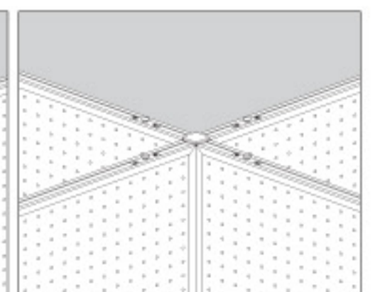
四方向連結(十字)
